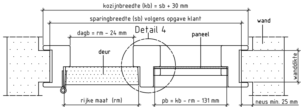
Doorsnede AA
