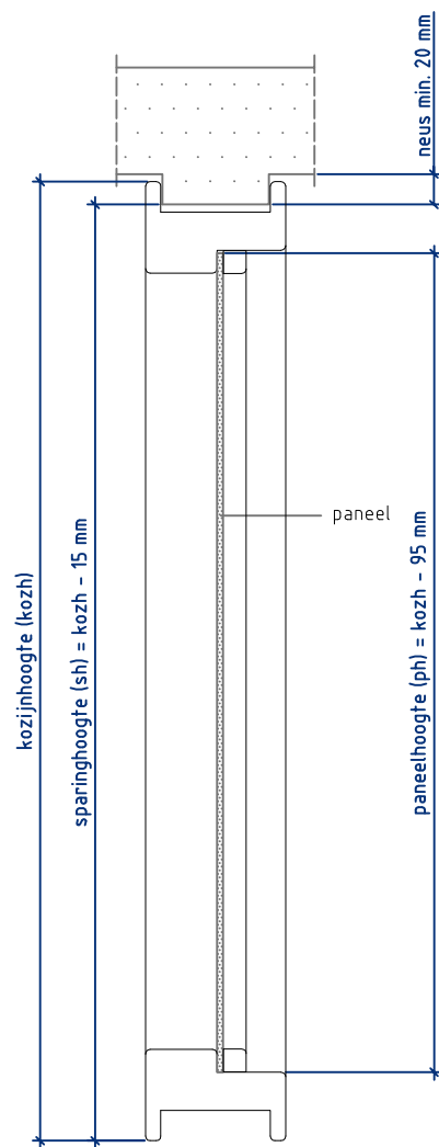
Doorsnede CC
