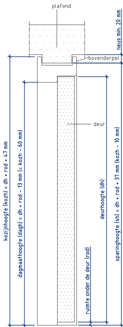
Doorsnede BB
