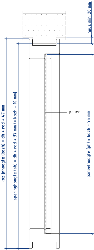
Doorsnede BB
