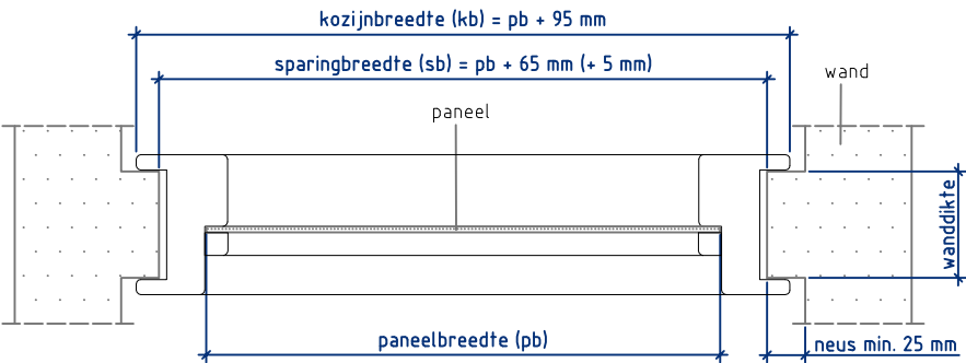
Doorsnede AA
