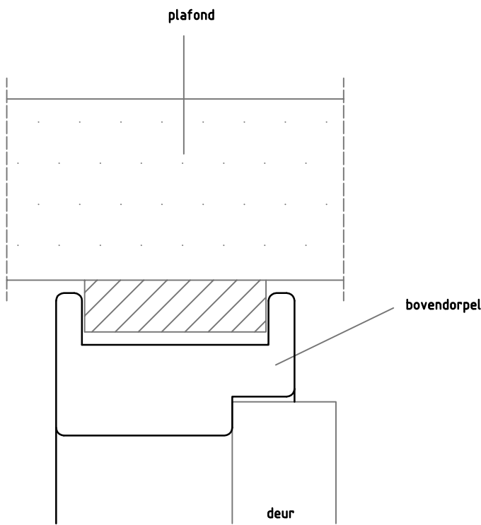
Detail 2: bovendorpel
