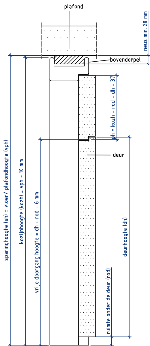
Doorsnede BB
