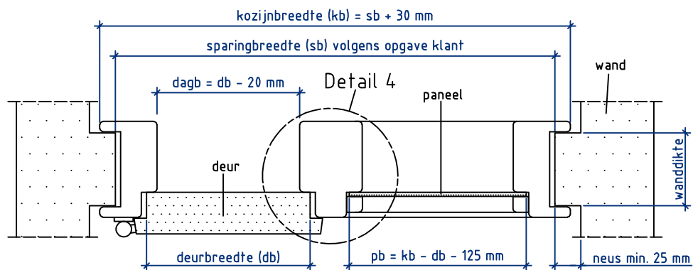
Doorsnede AA
