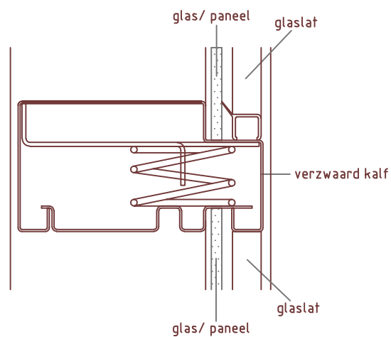
Detail 7: verzwaard kalf
