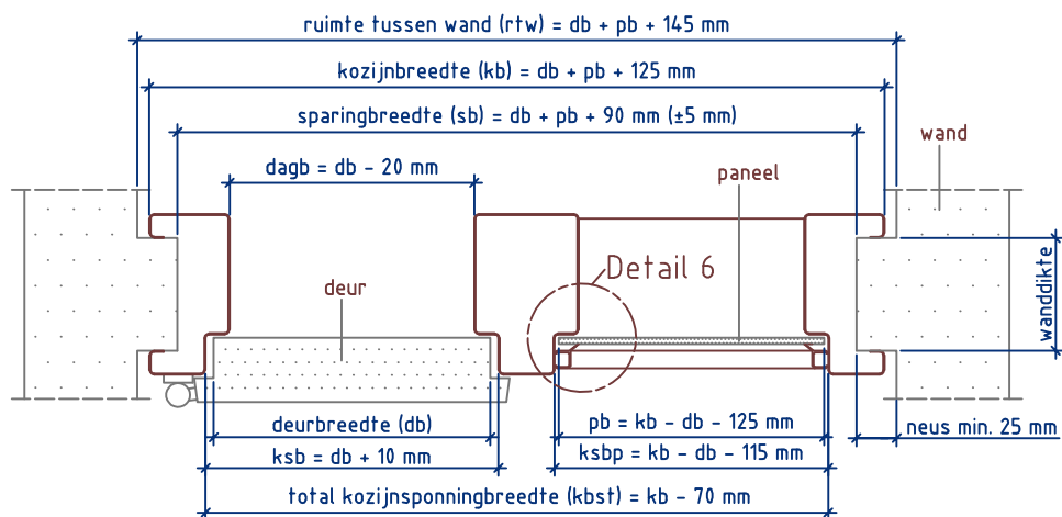
Doorsnede AA
