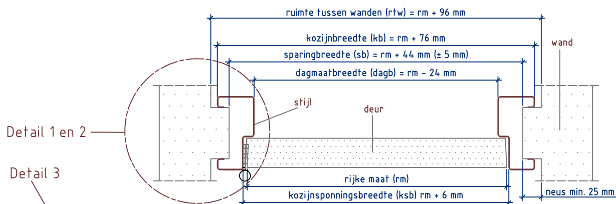
Doorsnede AA
