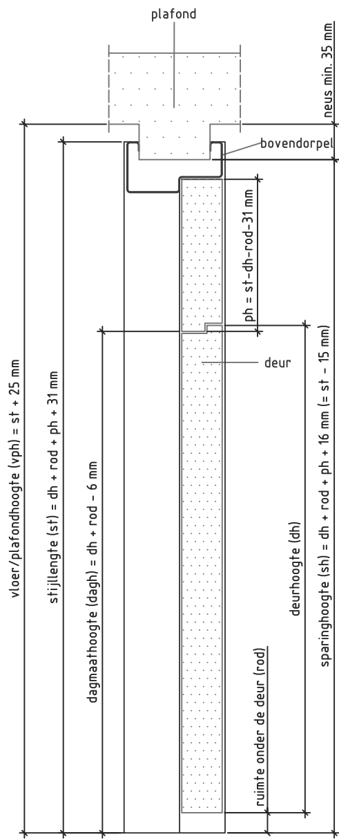
Doorsnede BB
