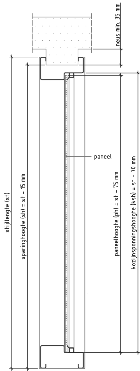
Doorsnede CC
