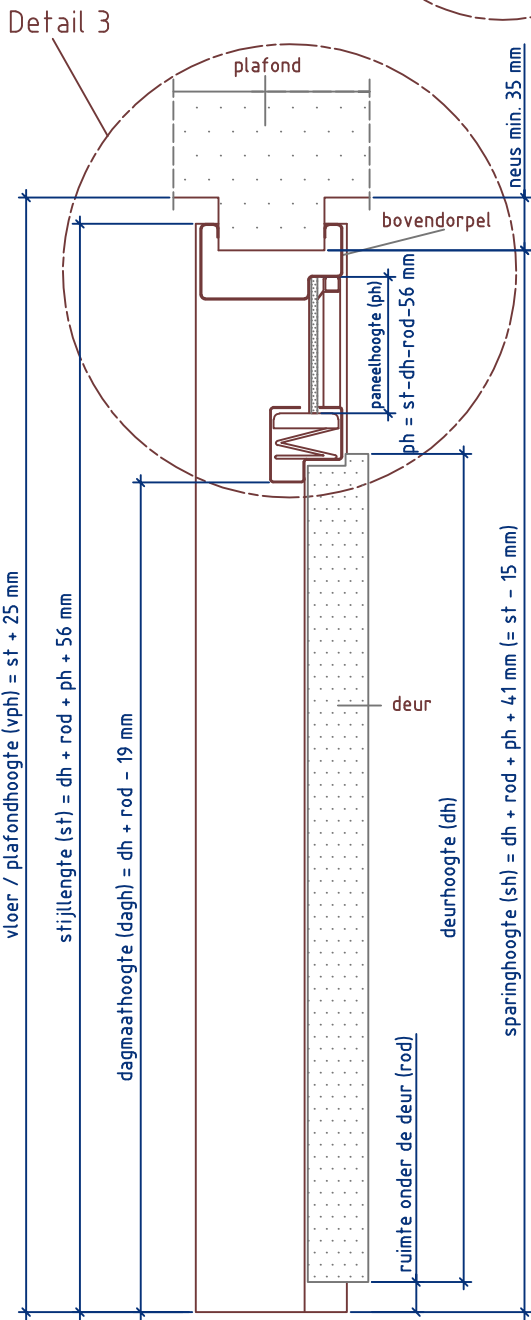
Doorsnede BB
