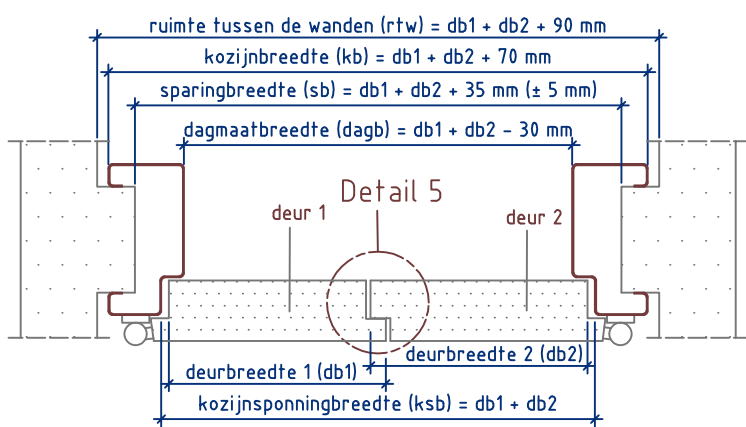
Doorsnede AA sponning/contrasponning
