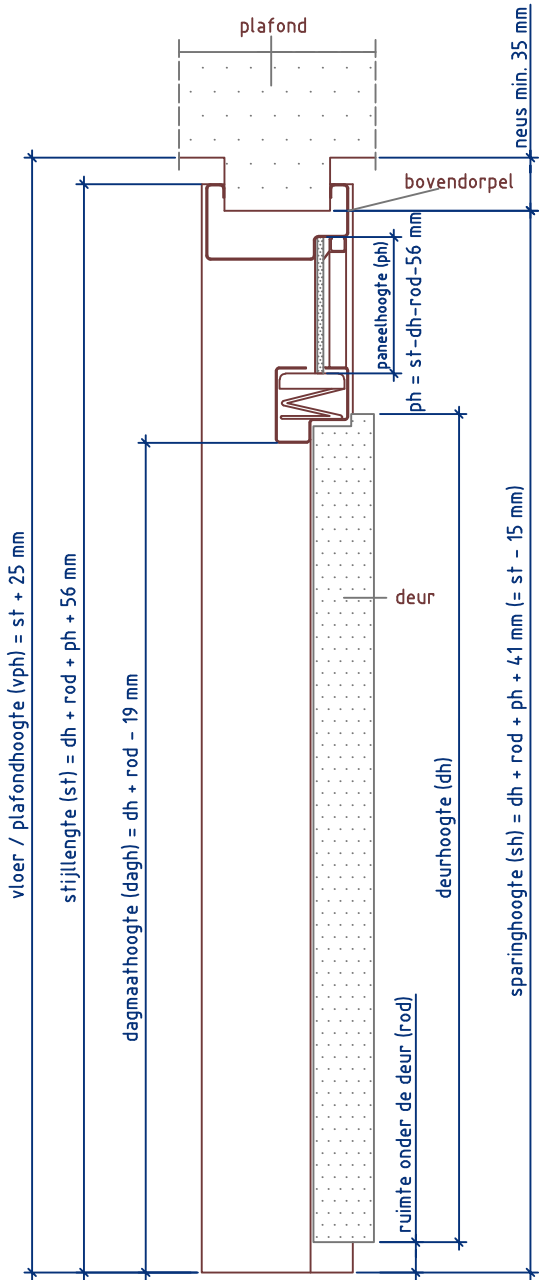
Doorsnede BB
