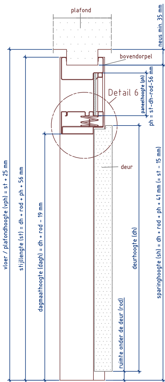
Doorsnede BB
