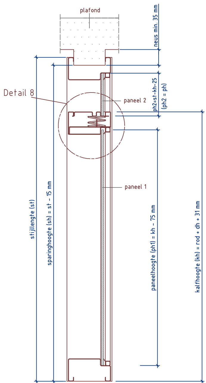
Doorsnede CC
