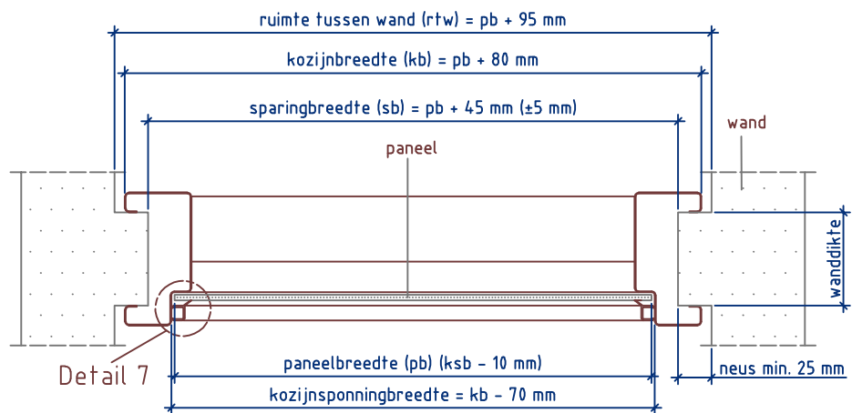
Doorsnede AA
