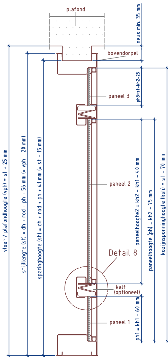
Doorsnede BB
