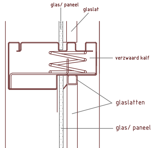
Detail 5: kalf zijlicht
