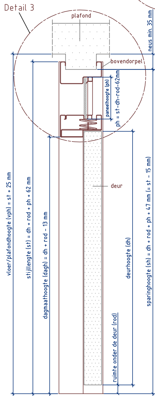
Doorsnede BB
