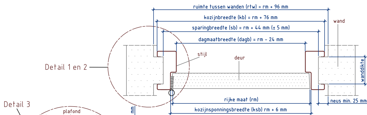
Doorsnede AA
