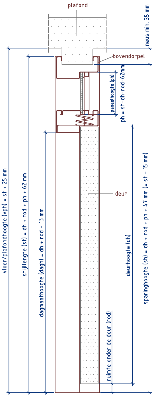
Doorsnede BB
