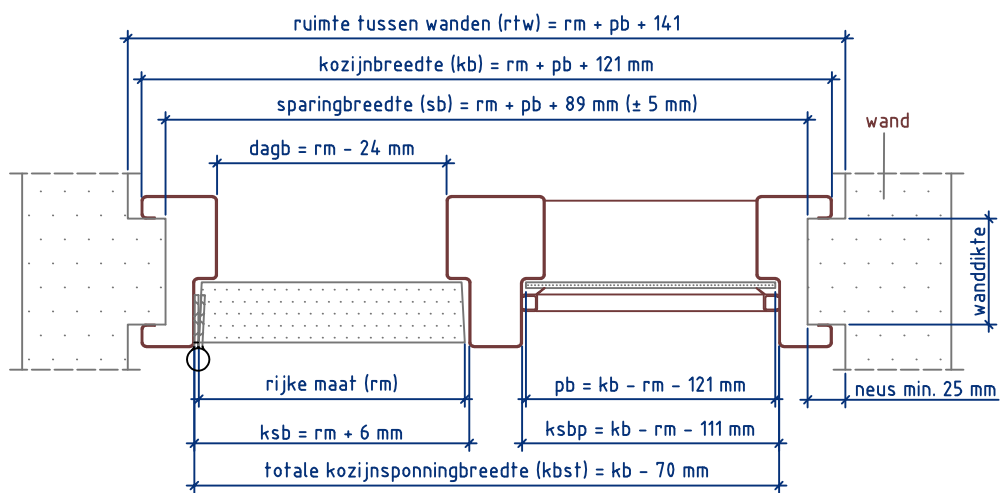
Doorsnede AA
