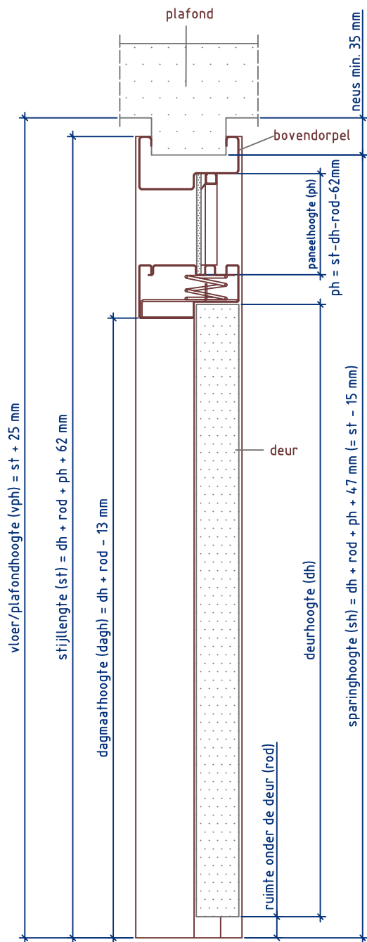
Doorsnede BB
