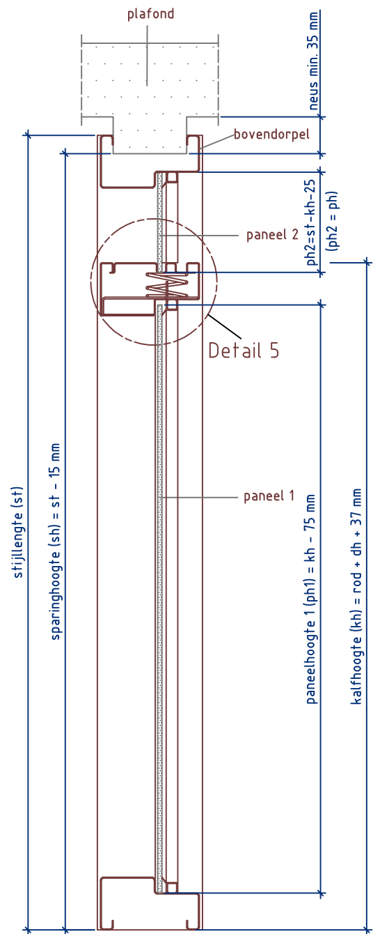
Doorsnede CC
