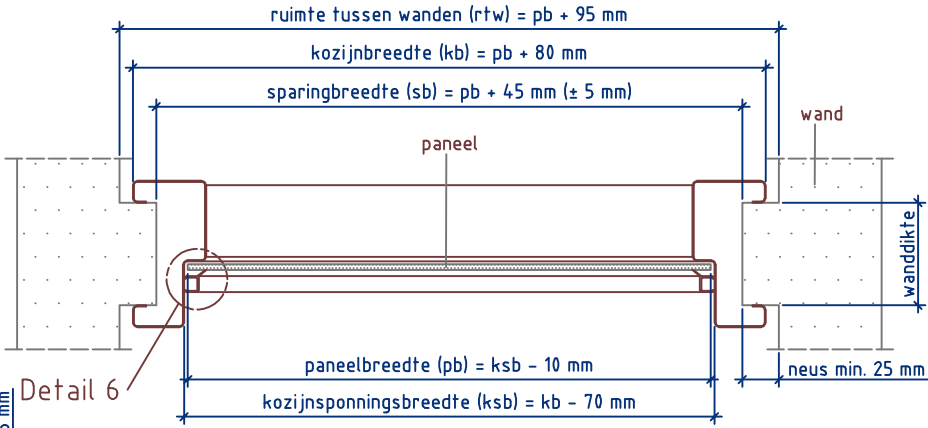
Doorsnede AA
