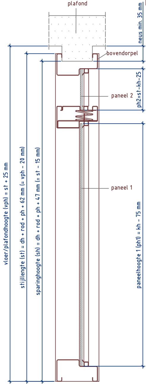
Doorsnede BB
