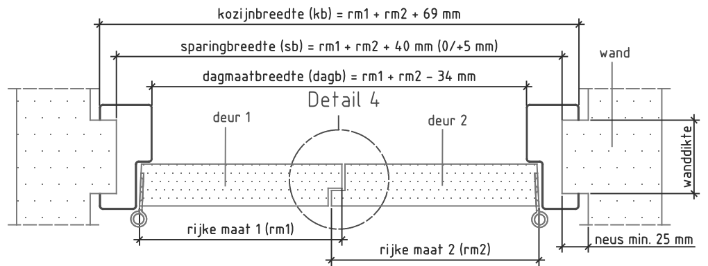
Doorsnede AA
