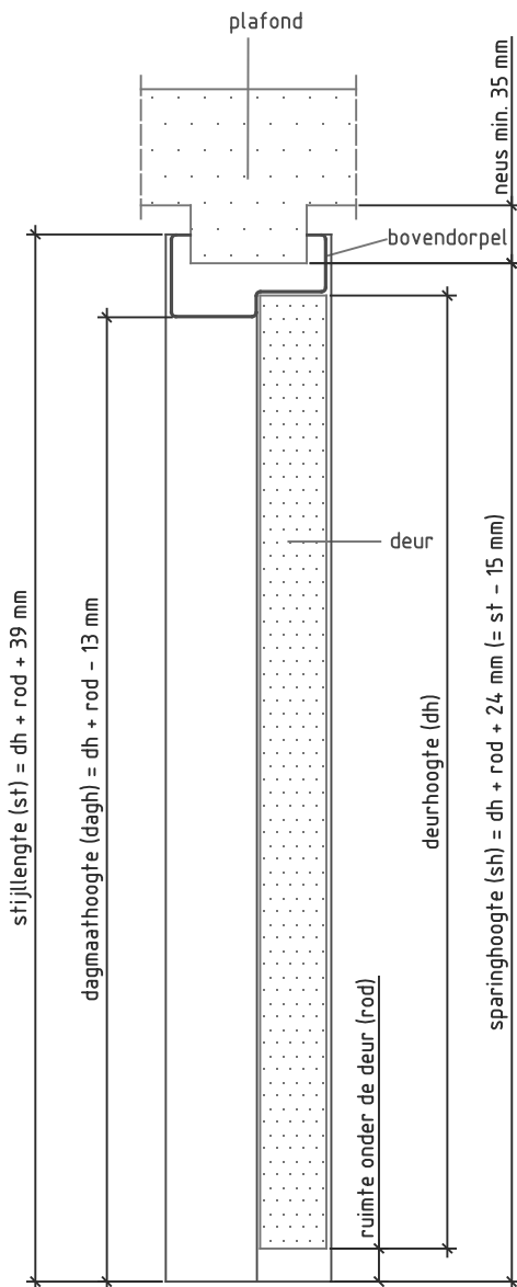
Doorsnede BB
