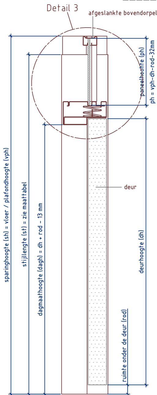
Doorsnede BB
