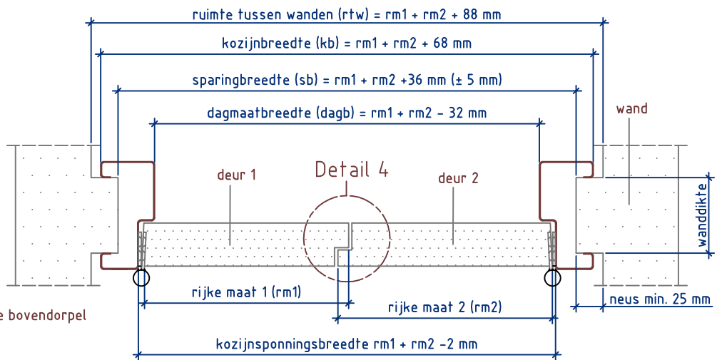
Doorsnede AA
