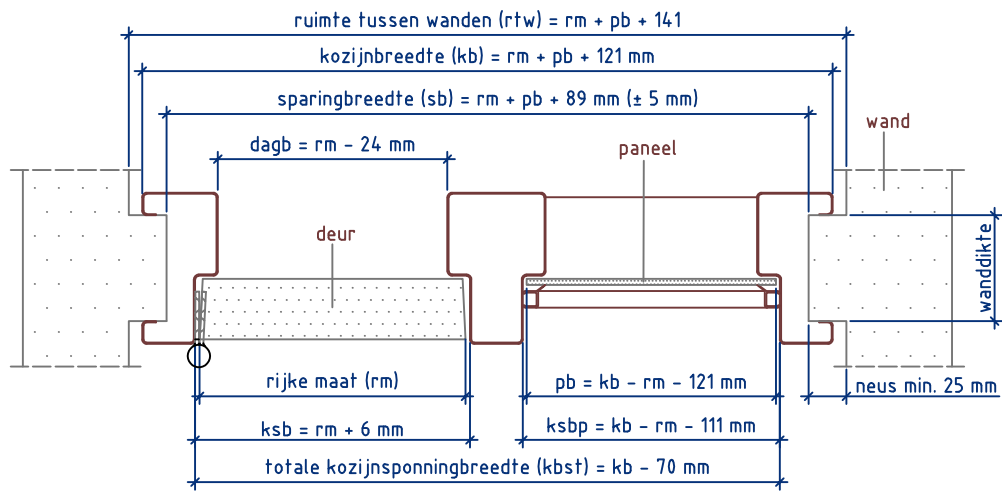
Doorsnede AA
