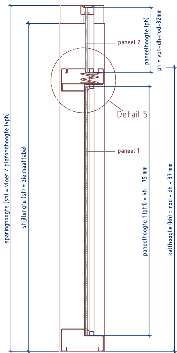
Doorsnede CC
