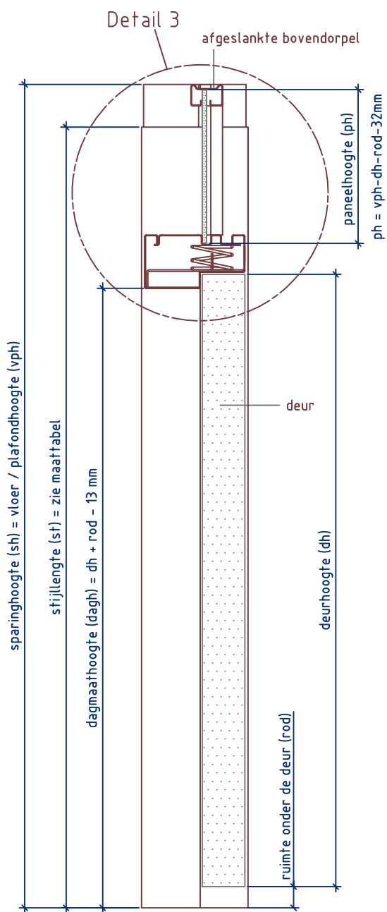
Doorsnede BB
