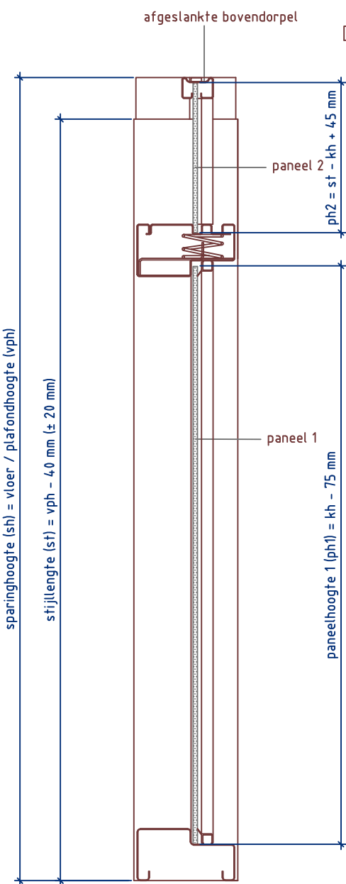
Doorsnede BB
