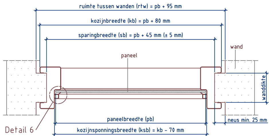
Doorsnede AA
