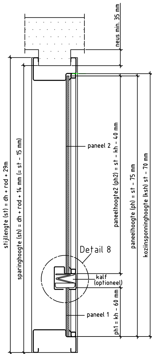
Doorsnede BB
