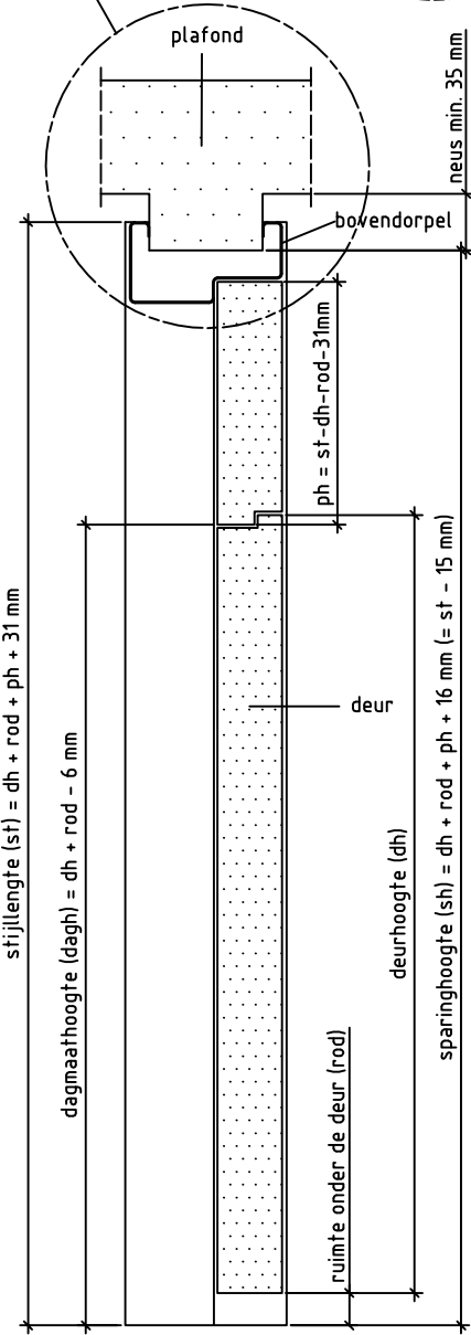
Doorsnede BB
