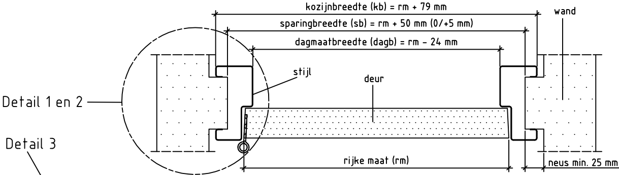
Doorsnede AA
