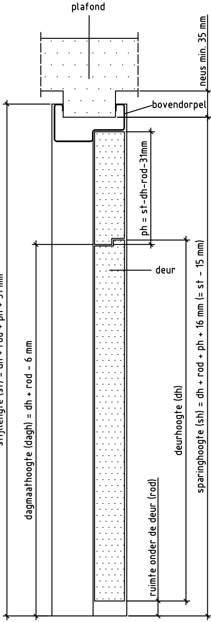
Doorsnede BB
