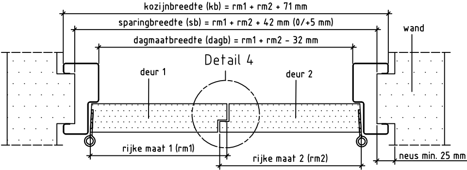
Doorsnede AA
