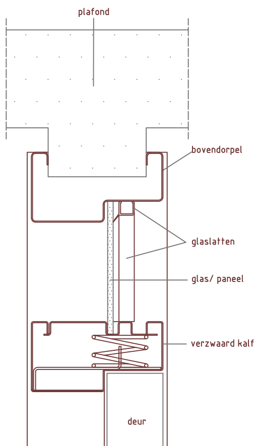
Detail 3: bovendorpel
