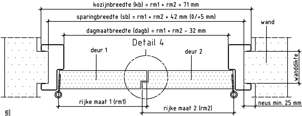
Doorsnede AA
