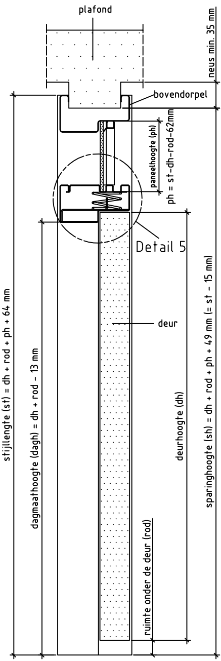
Doorsnede BB
