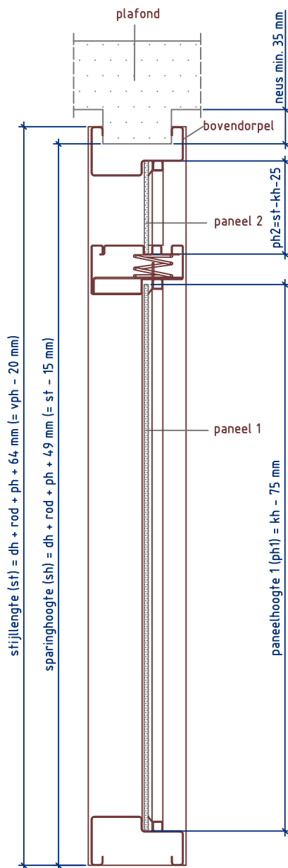
Doorsnede BB
