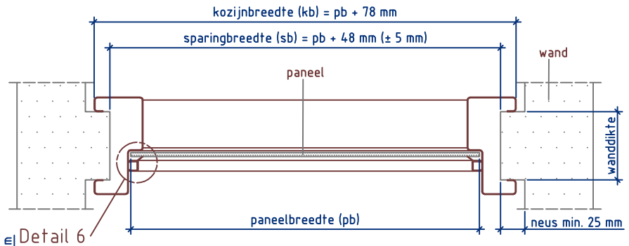
Doorsnede AA
