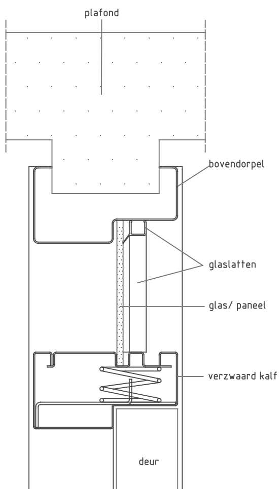
Detail 3: bovendorpel
