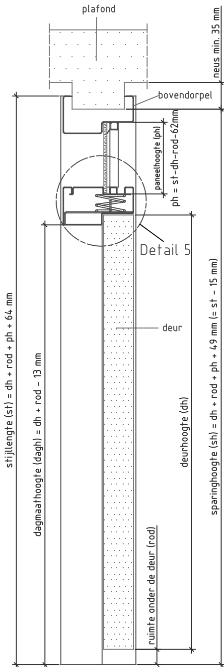
Doorsnede BB
