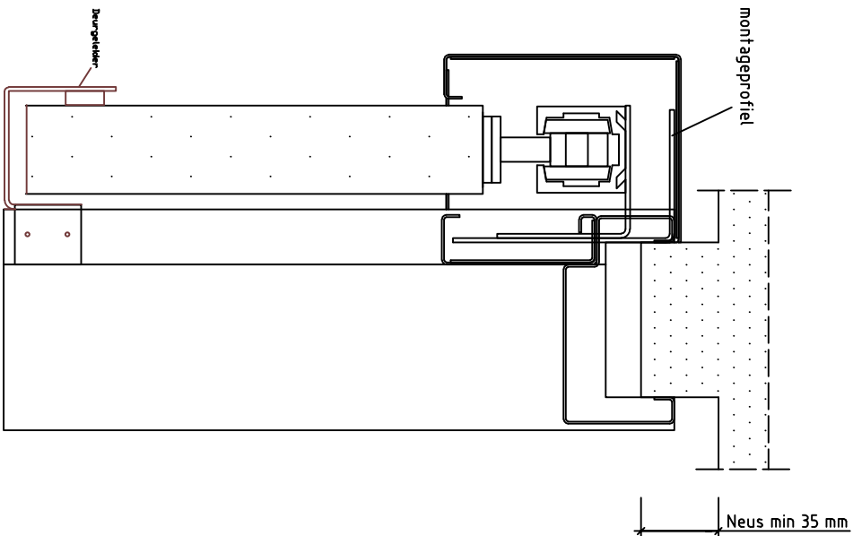
Doorsnede BB
